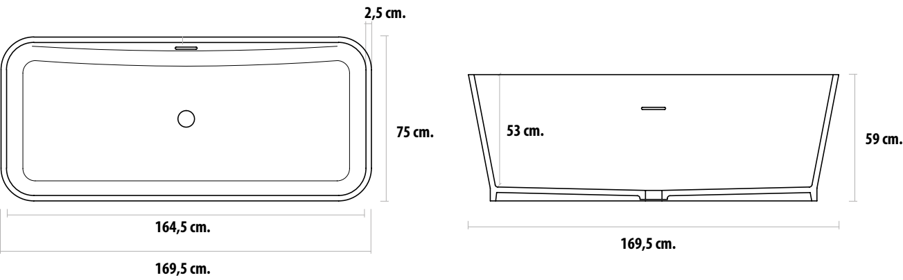
Bañera con rebosadero | Bathtubs with overflow | Baignoires à débordement | Vasche con troppo pieno.
